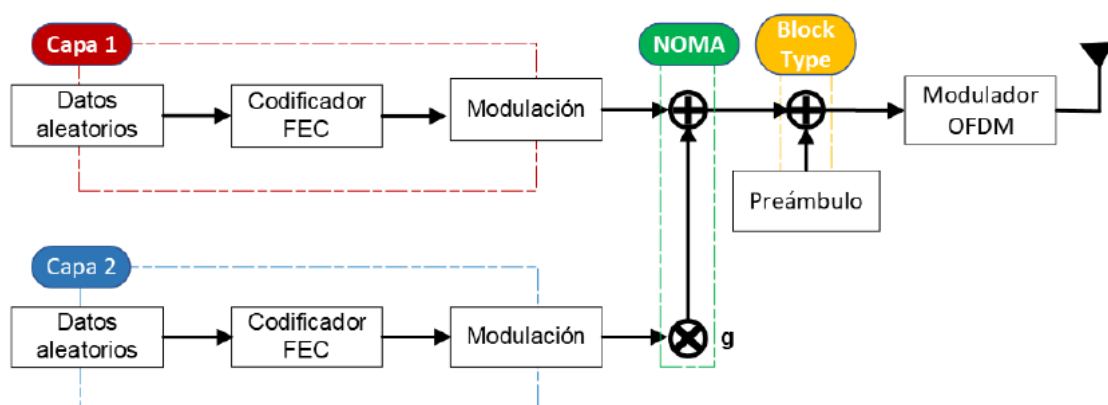
Figura 1. Diagrama de bloques del transmisor NOMA – OFDM.
