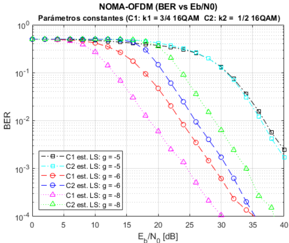
Figura 7. BER vs E_b/N_0 con estimación de canal LS para distintos valores de g .
