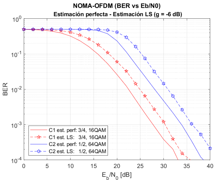
Figura 5. BER vs E_b/N_0 . Capa 1: tasa de codificación 3/4 y modulación 16QAM. Capa 2: tasa de codificación 1/2, modulación 64QAM y g de -6 dB.
