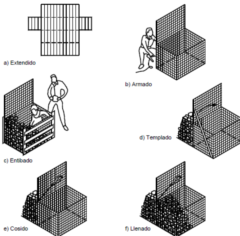
Ilustración 4 PROCESO CONSTRUCTIVO DE GAVIONES [9].
