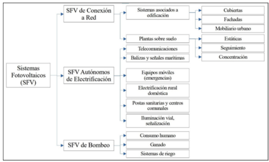
FIGURA 1 Clasificación de aplicaciones fotovoltaicas. Adaptado de Perpiñán (2020)
