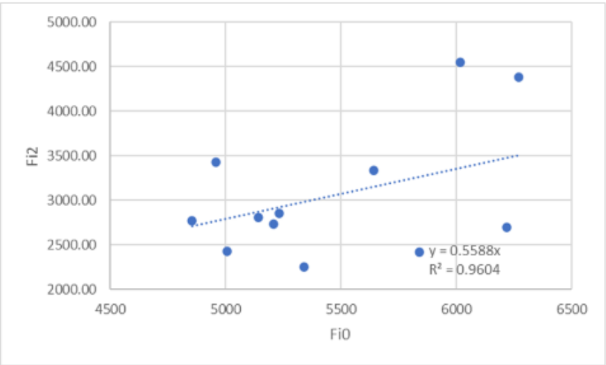
FIGURA 14. Regresión lineal Fi2.
