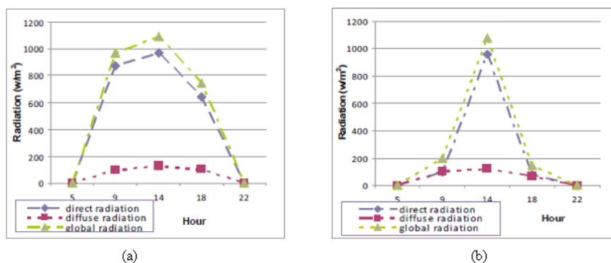
FIGURA 2. Radiación directa, difusa y global: (a) antes y (b) después de la arborización.
