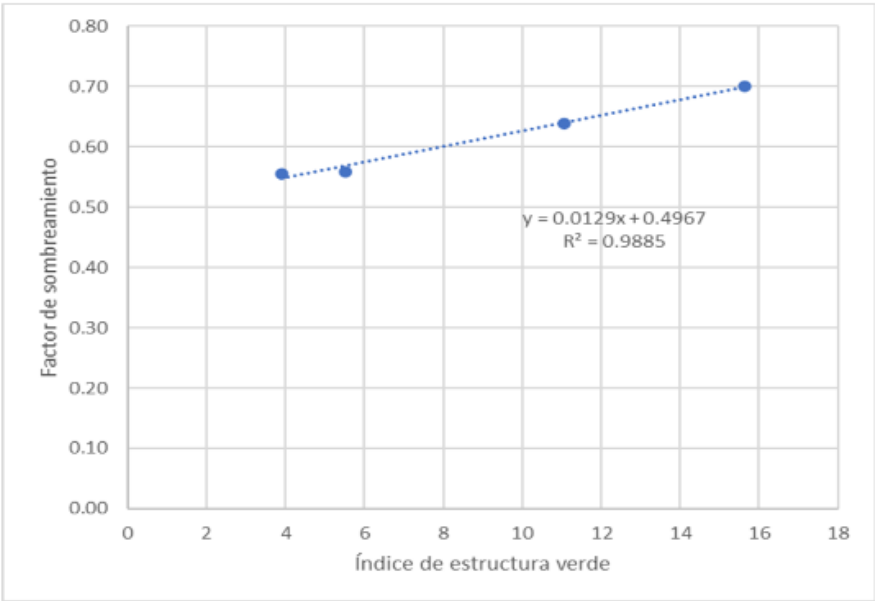
FIGURA 17. Regresión lineal entre factores de sombreamiento.
