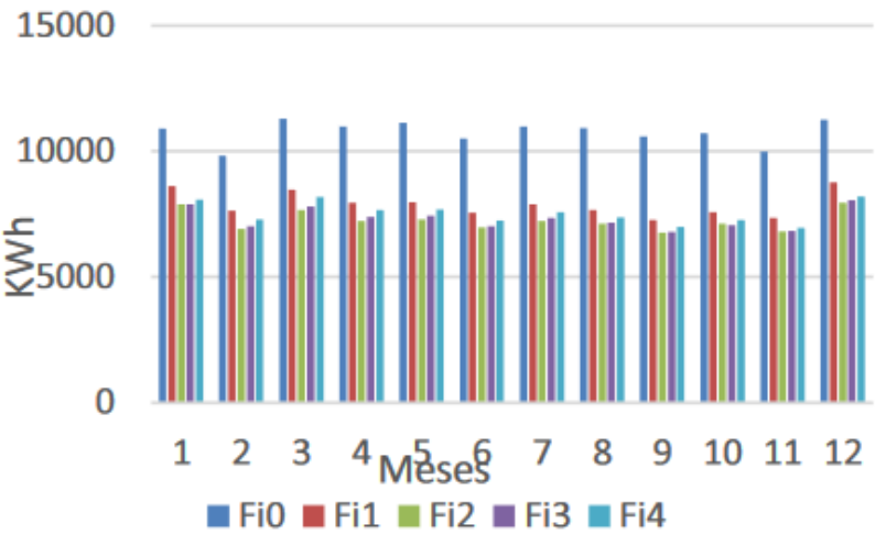
FIGURA 11. Comparativa entre los diferentes escenarios del edificio de apartamentos.
