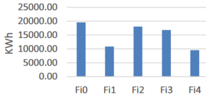
FIGURA 8. Ganancias solares por ventana edificio de apartamentos.
