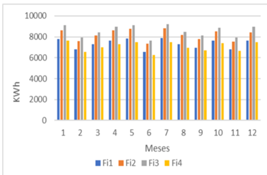
FIGURA 6. Consumo eléctrico edificio de oficinas.
