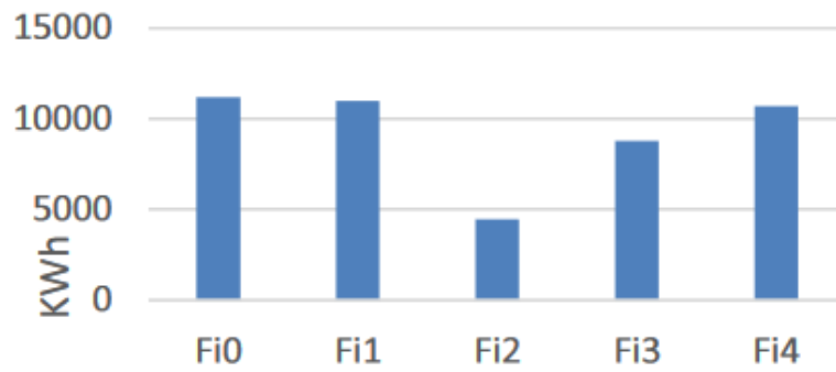
FIGURA 7. Ganancias solares anuales por ventana en el edificio de apartamentos.
