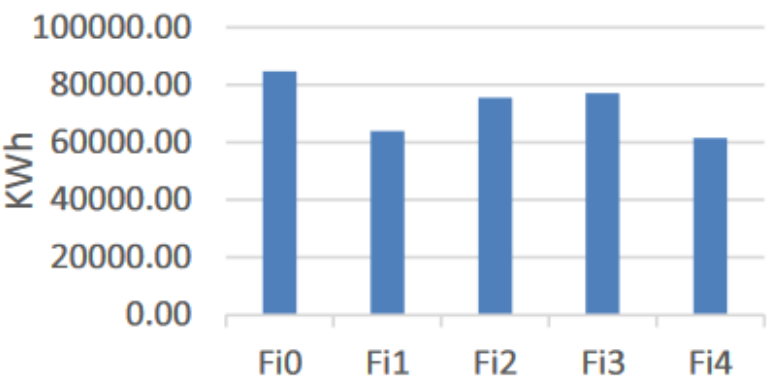
FIGURA 10. Ganancias solares por paredes edificio de oficinas.
