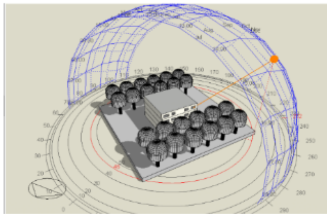
FIGURA 18. Escenario Fi5 del edificio de apartamentos para validación del modelo.
