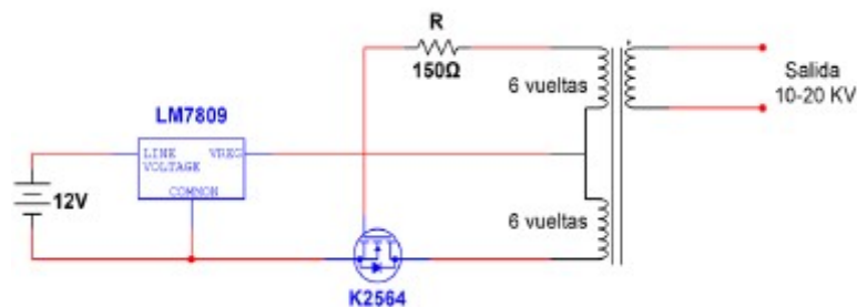
FIGURA 3. Esquema del circuito 2.
