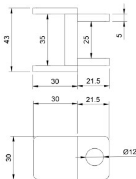
FIGURA 7. Esquema de soporte de perfil grueso (dimensiones en mm).
