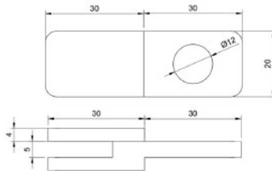
FIGURA 6. Esquema de soporte de perfil delgado (dimensiones en mm).
