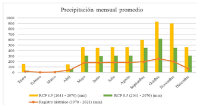
FIGURA 3. Comparación del registro histórico de precipitación mensual promedio y proyecciones de precipitación mensual promedio.
