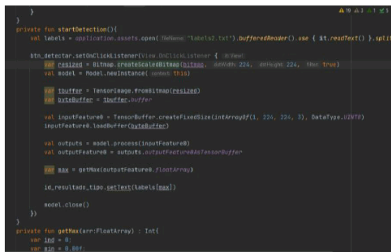
FIGURA 3. Uso de kotlin para la conexión de modelo TFLite .
