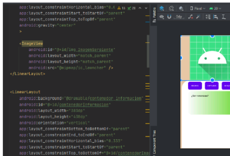
FIGURA 2. Uso de XML para la creación de las pantallas.
