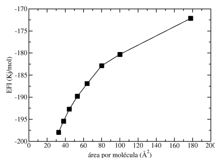
Figura 6: Energía para la formación de la interfaz de los sistemas vacío/SDS/agua en función del área por molécula.
