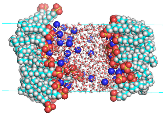
Figura 1: Sistema SDS/agua/SDS previamente relajados utilizando el programa Gromacs-4.5.5.
