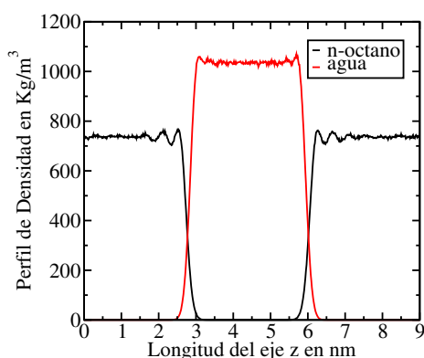
Figura 8: Perfil de densidad del sistema agua/n-octano obtenido con GROMACS 4.5.5.
