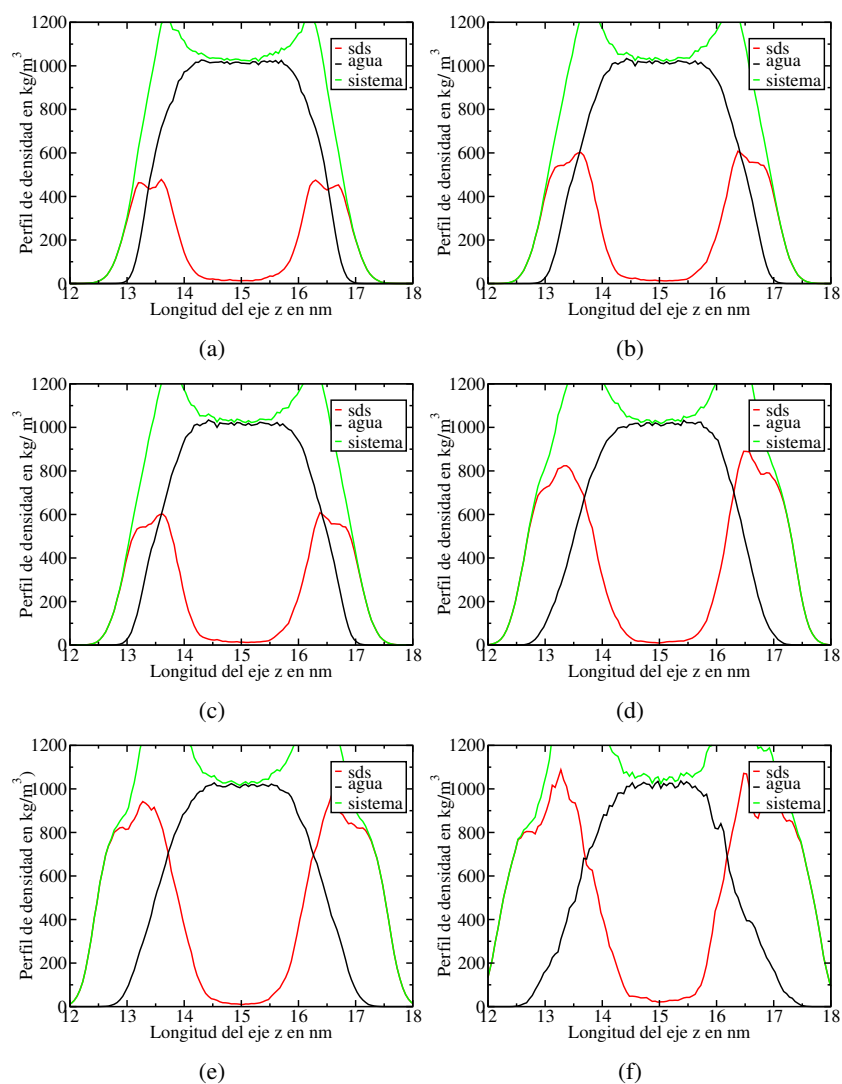
Figura 3: Perfiles de densidad de los sistemas SDS/agua/SDS. (a) 9 moléculas de SDS. (b) 12 moléculas de SDS. (c) 16 moléculas de SDS. (d) 20 moléculas de SDS. (e) 25 moléculas de SDS. (f) 30 moléculas de SDS.
