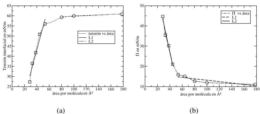
Figura 5: a) Tensión interfacial de los sistemas vacío/SDS/agua en función del área por molécula. b) Presión superficial de los sistemas vacío/SDS/agua en función del área por molécula.
