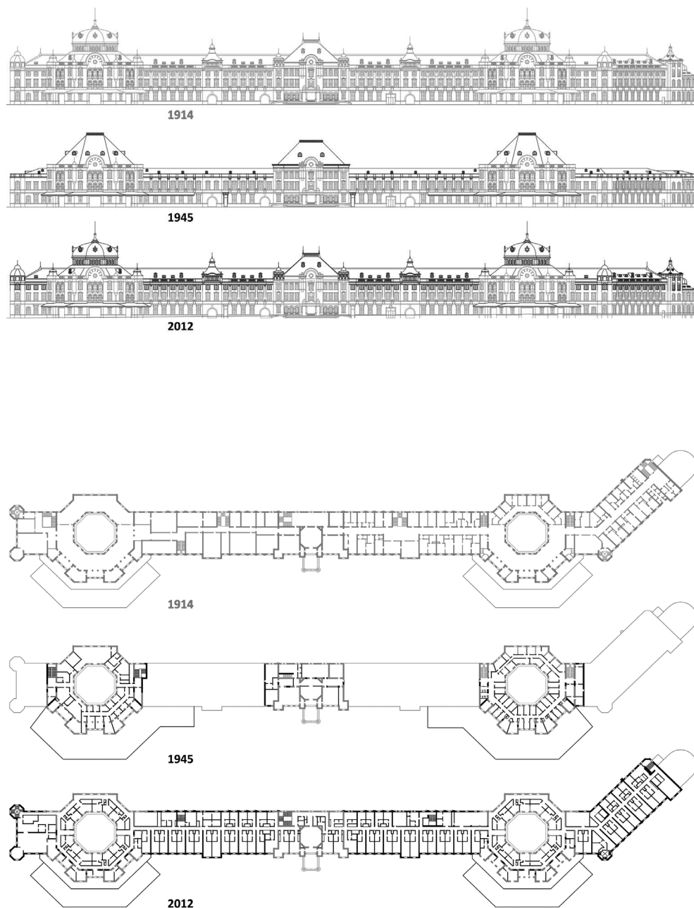
FIGURAS 9 E 10. PROCESSO DE TRANSFORMAÇÃO DO PISO 3: 1914 – edificação inicial; 1945 – demolição e construção da nova cobertura; 2012 – restituição da Estação à imagem inicial. Imagem: José Miguel Silva.
