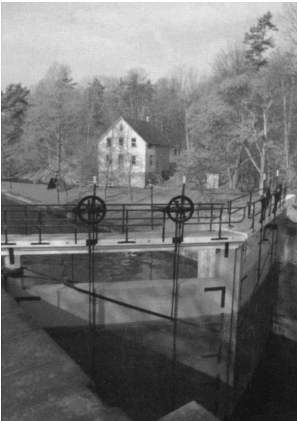
CANAL RIDEAU. La autenticidad de los canales en funcionamiento en el Canal Rideau, un canal histórico canadiense inscrito en la Lista de Patrimonio Mundial en 2007, se basa en la conservación de las formas originales de diseño más que del material de madera original, ahora deteriorado y reemplazado muchas veces. Imagen: Herb Stovel.
