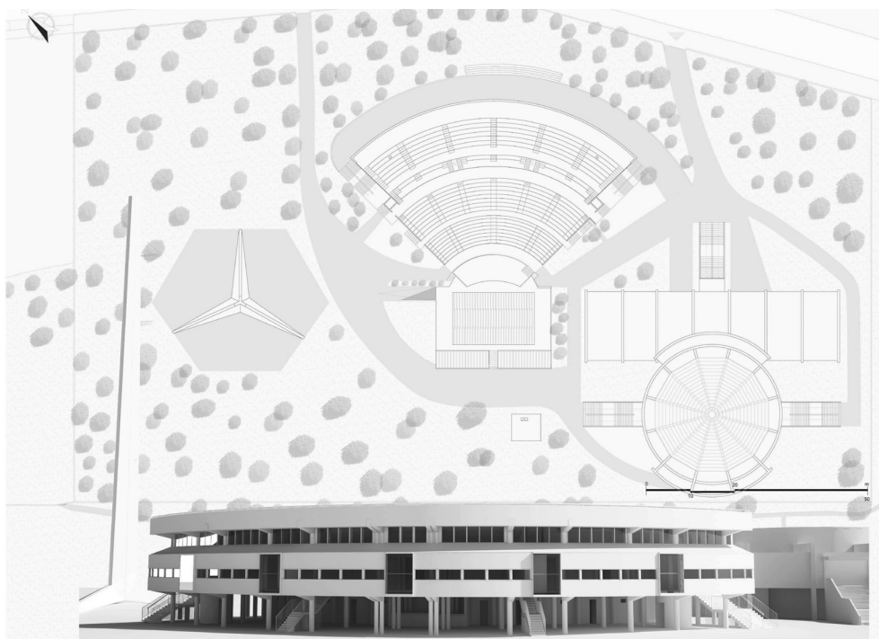
FIGURA 6. RILIEVO DELLA PIANTA PIANO TERRA E DEL PROSPETTO PRINCIPALE.
