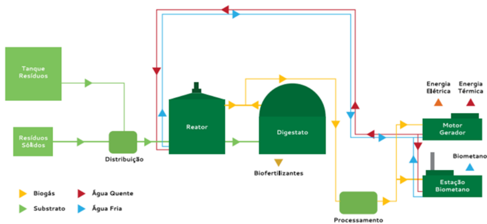
Figura 1. Diagrama básico de la Planta de Biogás del Proyecto Concordia/SC. Fuente: (Probiogás, 2015).
