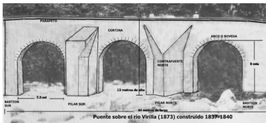
FIGURA 1 Elementos estructurales del puente sobre el río Virilla Fuente: Elaboración propia a partir de la fotografía 1.
