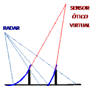
FIGURA 2 definição de uma geometria equivalente ótica Fonte: autor (2023)
