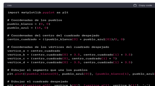
Figura 22. Código Python devuelto por ChatGPT
