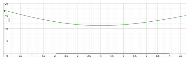
Figura 18. Representación gráfica de la función tiempo y su dominio
