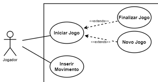
Figura 2. Diagrama de Casos de Uso do jogo
