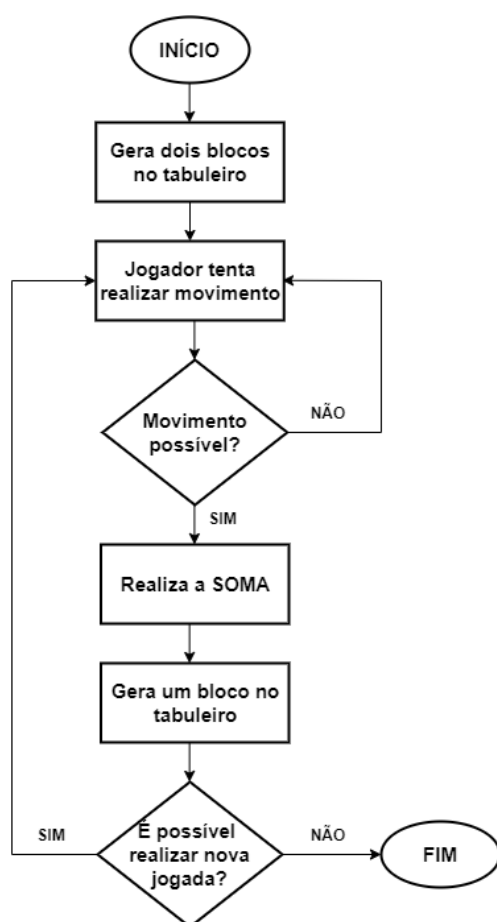
Figura 3. Fluxograma do jogo
