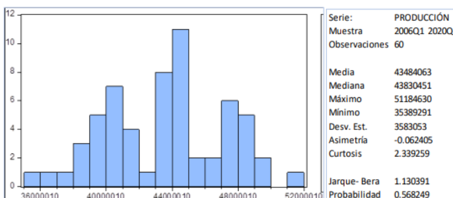
FIGURA 9 Prueba de normalidad Elaboración propia.
