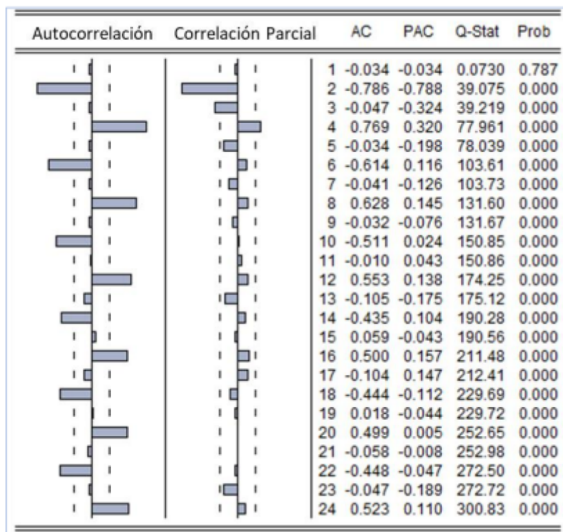
FIGURA 6 Correlograma para la serie dlog producción de leche Elaboración propia.
