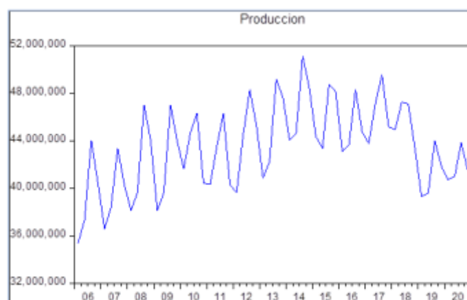
FIGURA 3. Gráfico de producción de leche en diferenciado y en logaritmo
