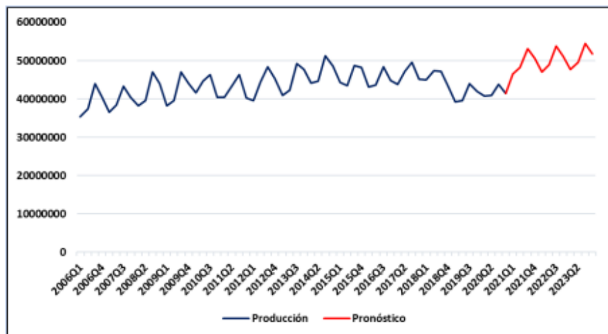
FIGURA 11. Pronóstico dinámico usando Ar (4) Ma (2) Ma (4) Ma (6) Elaboración propia.
