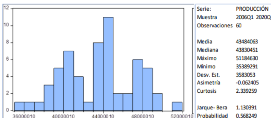
FIGURA 5. Prueba de normalidad
