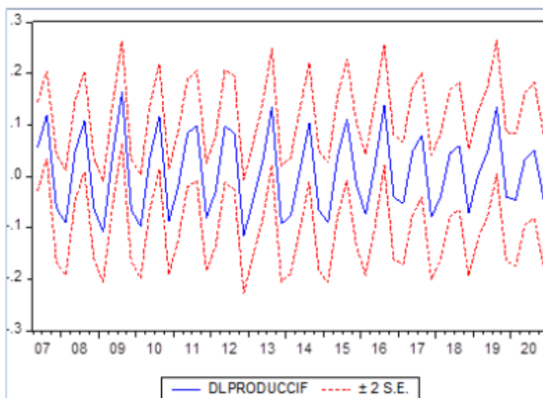
FIGURA 10 Pronóstico estático usando Ar(4) Ma(2) Ma(4) Ma(6) Elaboración propia.
