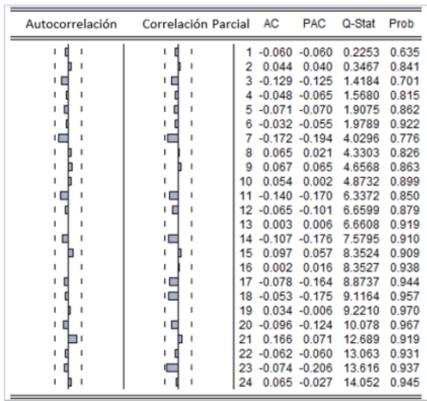
FIGURA 8. Validación de supuesto: correlograma de los residuos al cuadrado El autor con datos del INEC.
