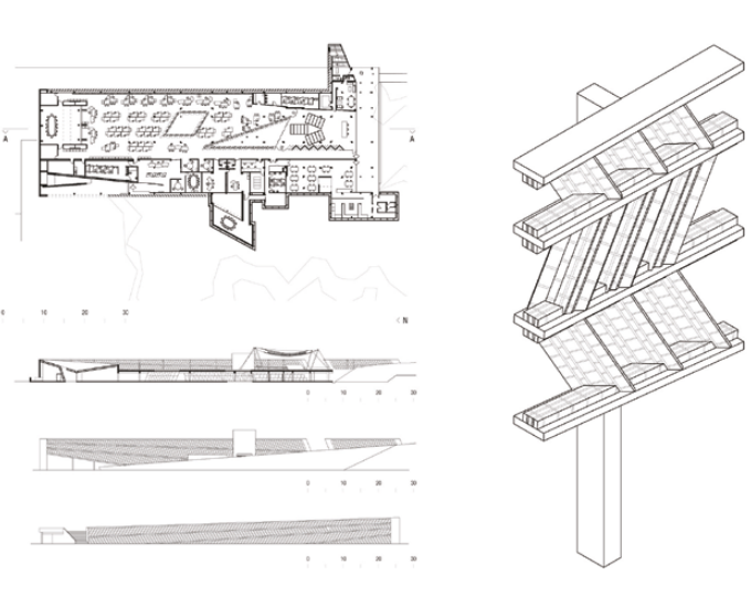
Figura 6. Celosía en la fachada de Unilever Paraguay (2000-01). Fuente: Enrico Cano ( www.enricocano.com/solano-benitez ). | Figura 7. Planta baja, sección longitudinal, fachadas y detalle de la celosía del edificio Unilever Paraguay (2000-01). Fuente: Dibujos de la autora.
