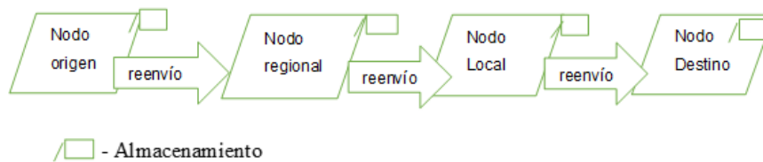
FIGURA 1 Esquema de mecanismo de transmisión de datos con DTN Elaborado con base en Romero y Sánchez (2010).
