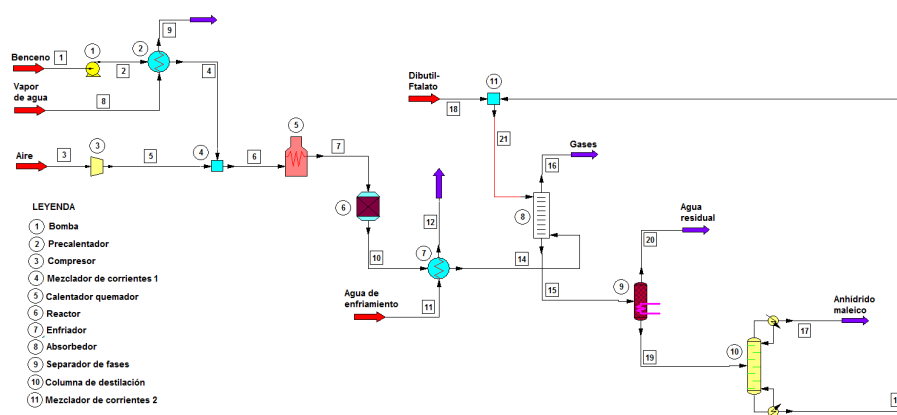
FIGURA 2. Diagrama de flujo del proceso de producción de AM a partir de benceno obtenido en el simulador ChemCADâ Fuente: elaboración propia.
