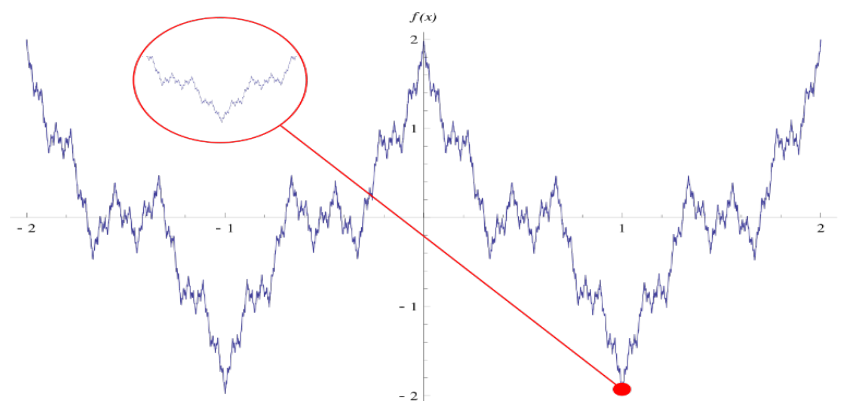
Figura 1 - Função de Weierstrass
