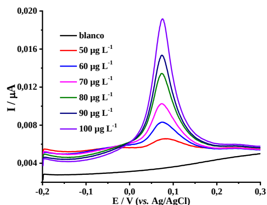
Figura 5. DPASV para diferentes concentraciones de \text{Hg(II)} . A 10 \text{ mV s}^{-1} , 0,8 \text{ V} en la preconcentración de \text{Hg} y -0,1 \text{ V} de electrodeposición de oro
