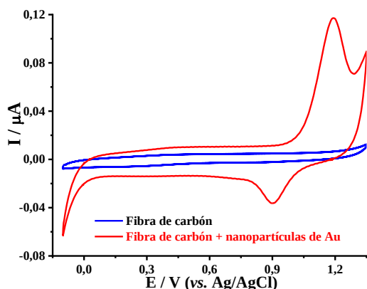
Figura 4. Voltamperograma de la microfibras de carbono sin modificar y modificada con nanopartículas de oro, en 0,05 \text{ mol L}^{-1} de \text{H}_2\text{SO}_4 , a v = 100 \text{ mV s}^{-1}
