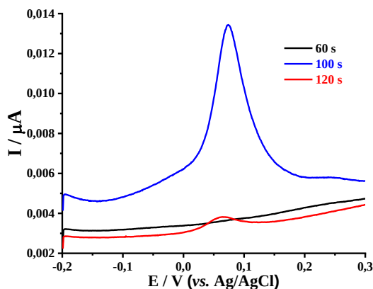
Figura 2. Detección de 80 \mu\text{g L}^{-1} \text{Hg(II)} , mediante DPASV, en la microfibras de carbono modificado con oro electrodepositado a diferentes tiempos
