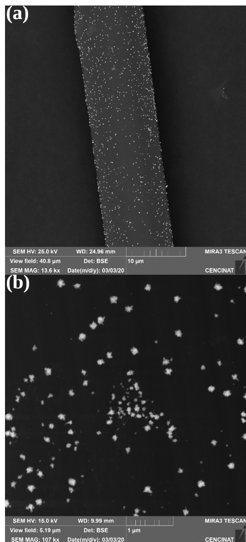
Figura 3. Imagen SEM de la microfibras de carbono modificado con nanopartículas de oro: (a) a 13,6 kx de ampliación, (b) a 107 kx
