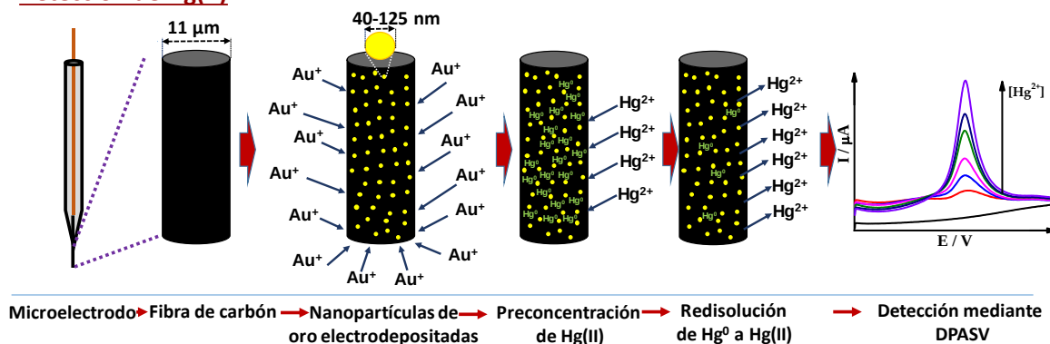
Figura 1. Construcción del microelectrodo de fibra de carbono y detección de \text{Hg(II)} por voltametría de redisolución anódica de pulso diferencial, adaptado de Carrera et al. (2017).
