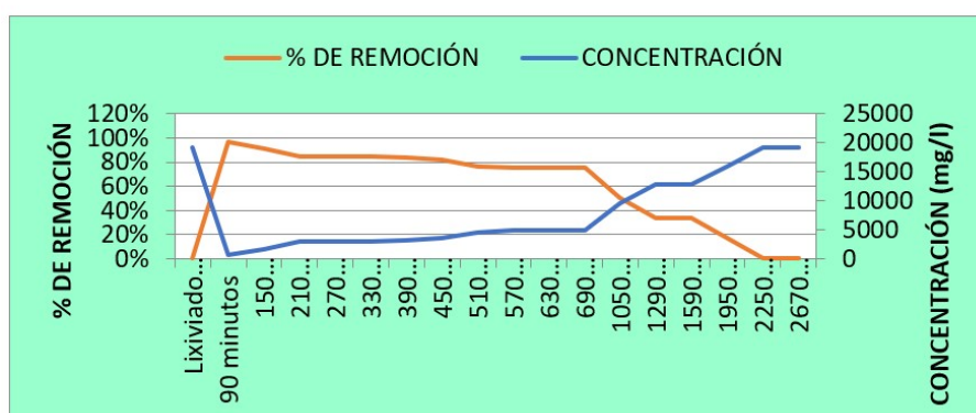
FIGURA 8. Eficiencia remoción de materia orgánica. pH 3,0. Autores
