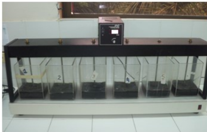
FIGURA 2. Reactor discontinuo. Autores
