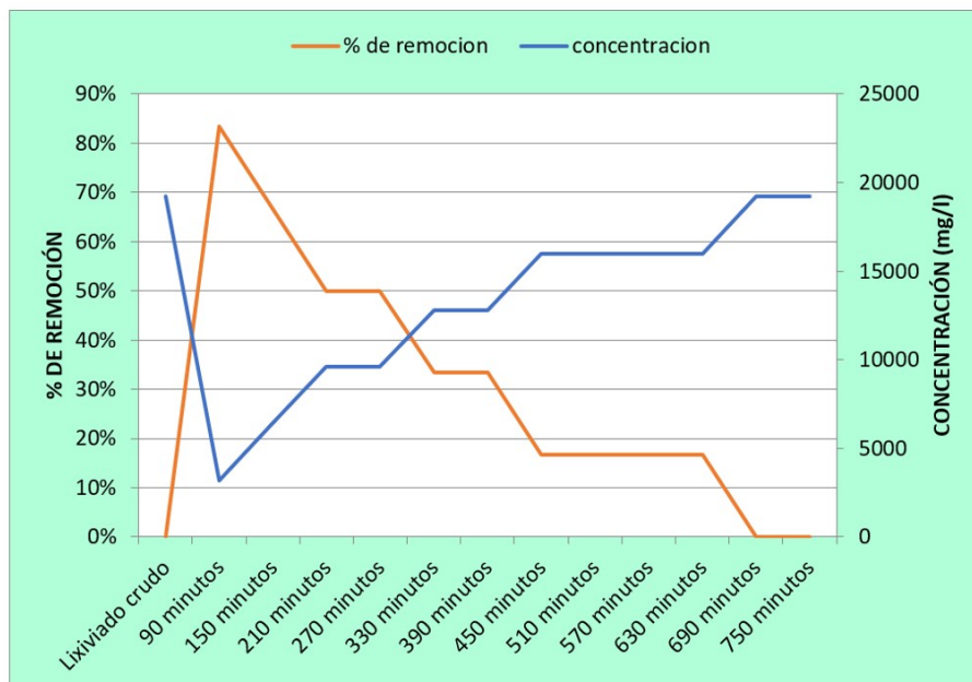
FIGURA 6. Eficiencia remoción de materia orgánica. PH lixiviado crudo. Autores
