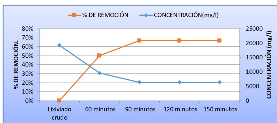
FIGURA 5. Eficiencia de remoción de DQO. Tiempo, pH de la muestra. Autores
