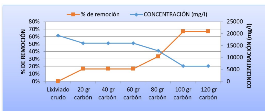
FIGURA 4. Eficiencia de remoción de DQO. Dosis, pH de la muestra. Autores
