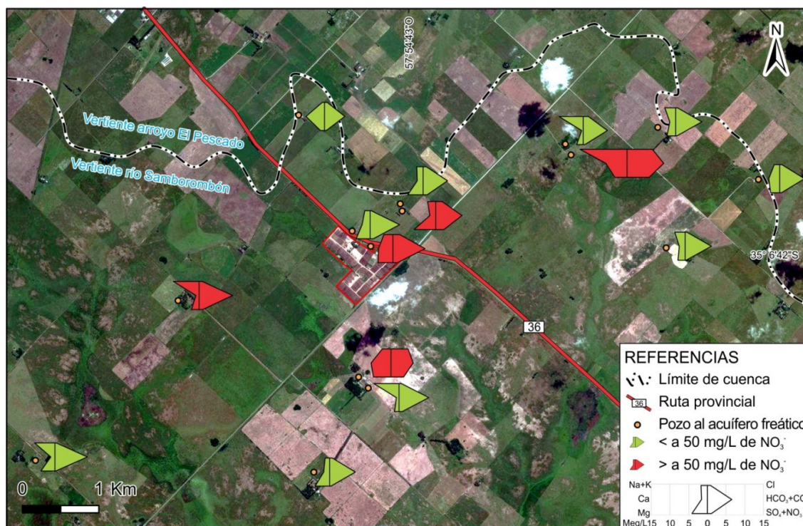
Figura 2. Diagramas de Stiff mostrando el contenido de iones mayoritarios de los puntos muestreados. En color rojo se indican las muestras que superan el límite de potabilidad del nitrato de la OMS (2008).
