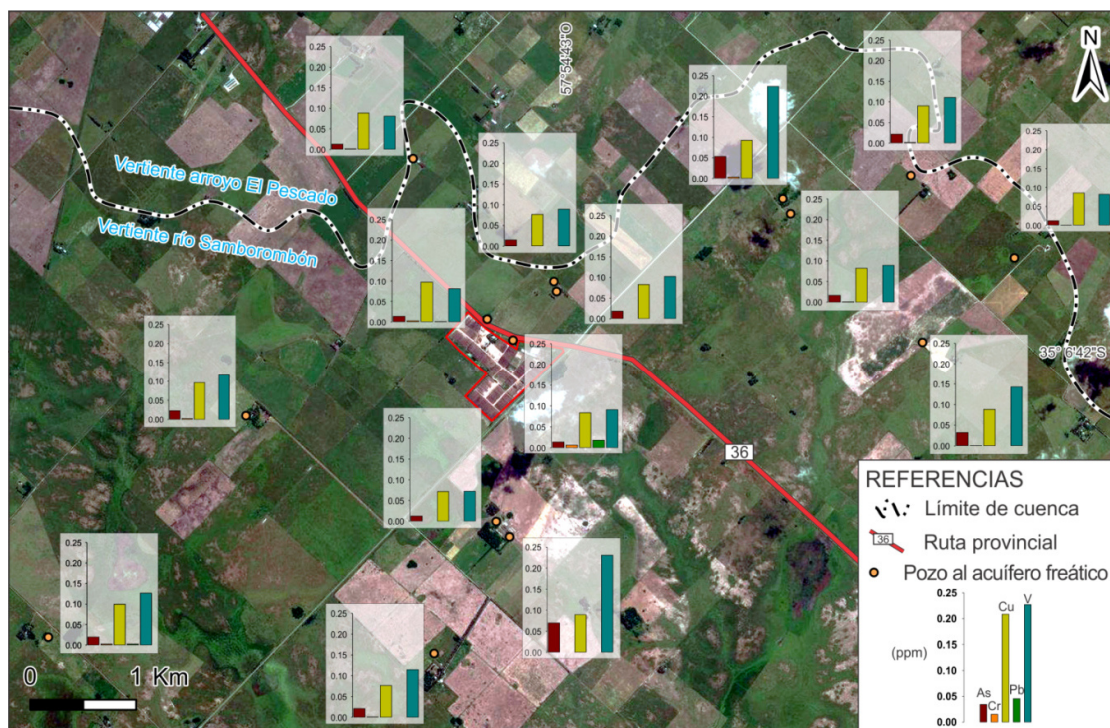
Figura 3. Contenido de elementos traza en el agua subterránea de los distintos puntos muestreados.
