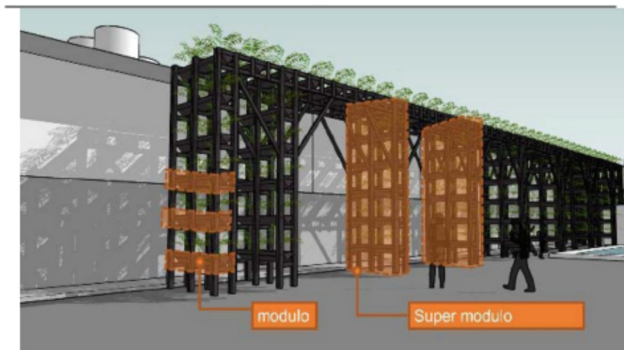
FIGURA 1. Vistas de la modulación de la Eco- fachada.
