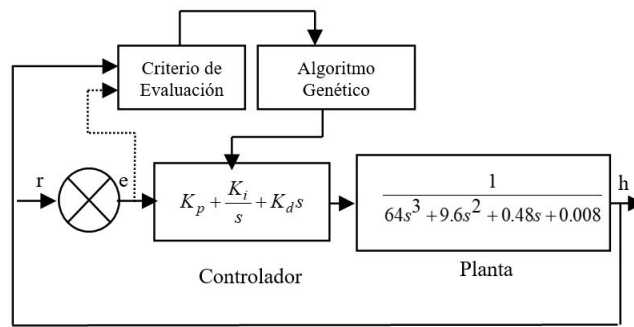
FIGURA 6 Figura 6: Planta con controlador PID genético.
