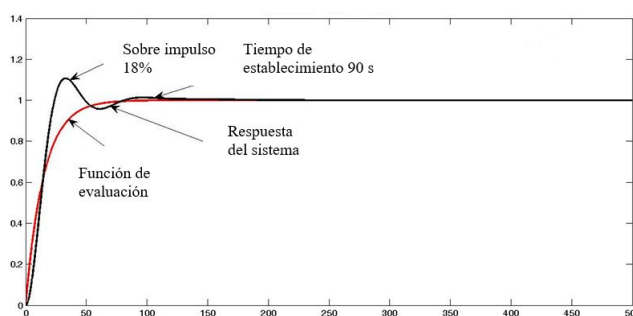
FIGURA 8 Figura 8: Planta con controlador PID genético.
