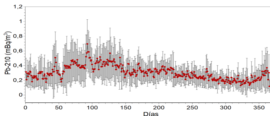
FIG. 13 Contenido promedio diario de Pb-210, en función del día del año (2006 al 2019)
