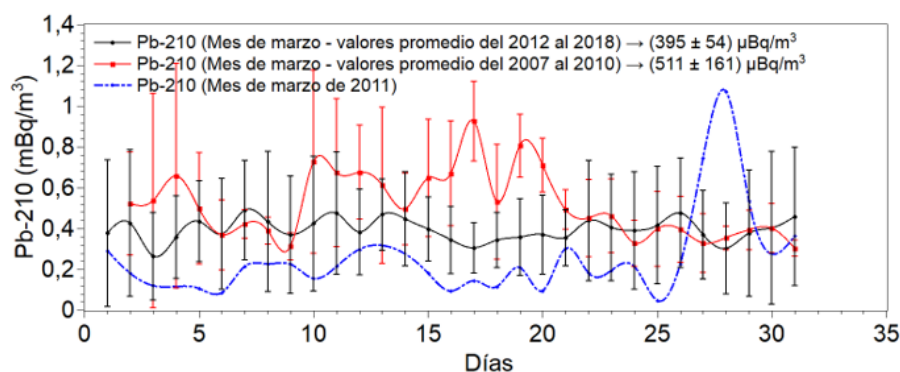
FIG. 16 Valores del Pb-210 durante el evento de Fukushima
