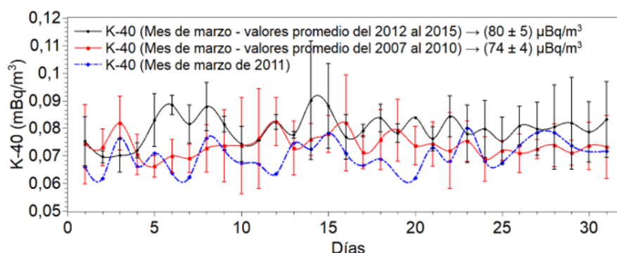
FIG. 17 Valores del K-40 durante el evento de Fukushima
