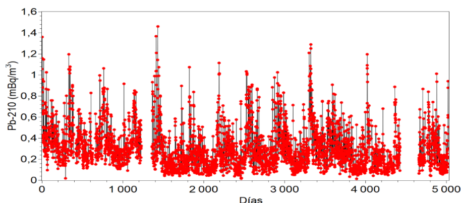
FIG. 12 Medición diaria del Pb-210 de 2006 a 2019
