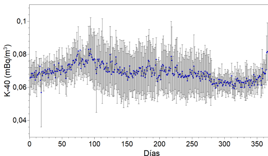
FIG. 10 Promedio diario del K-40 del 2006 al 2019
