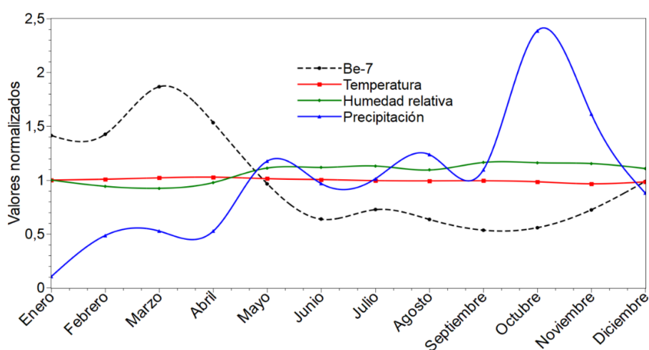
FIG. 4 Valores normalizados, por mes, de Be-7, Temperatura, Humedad, Precipitación del 2006 al 2019 (14 años de datos)
