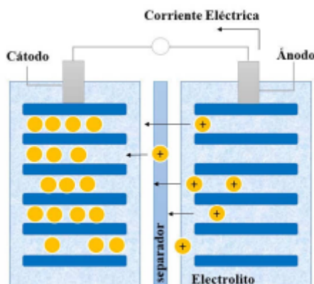
FIGURA 1. Partes de una batería
