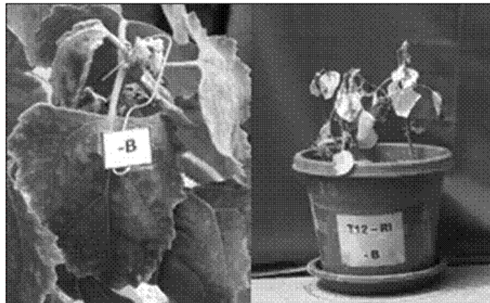
FIGURA 5 Síntomas de deficiencia de boro en plantas de quinua.
