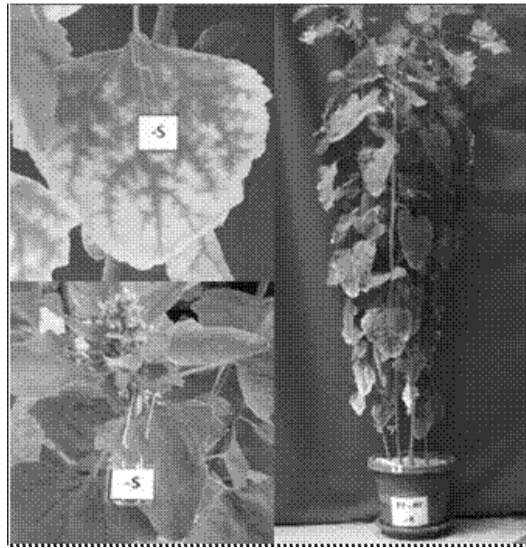
FIGURA 4 Síntomas de deficiencia de azufre en plantas de q
