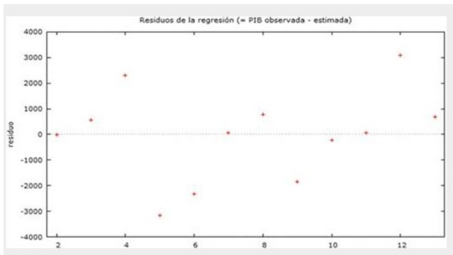
FIGURA 1 Gráfico de residuales obtenido con Gretl
