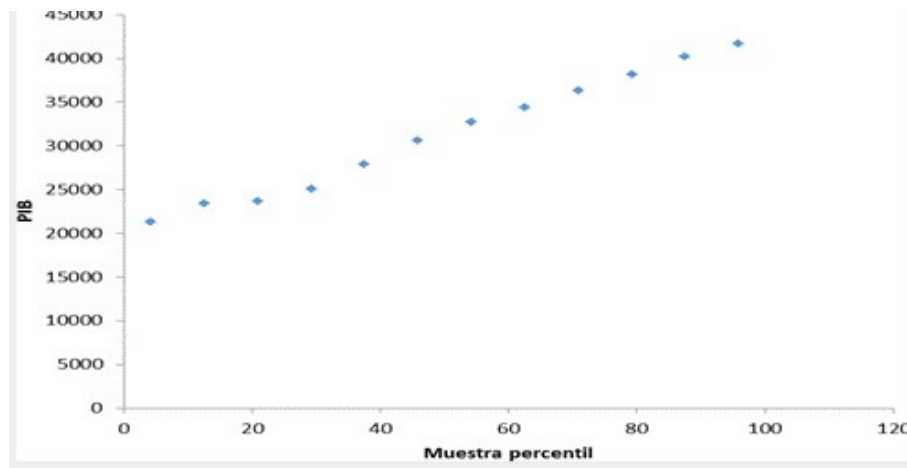
FIGURA 2. Gráfico de probabilidad normal a partir del programa Excel
