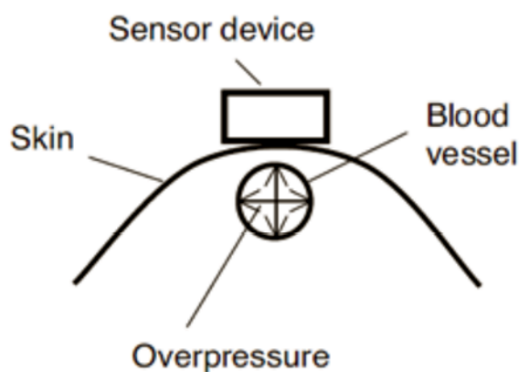
Fig. 11 Principio de monitoreo de presión arterial debido al desplazamiento de superficie (Kirstein et al. 2005)
