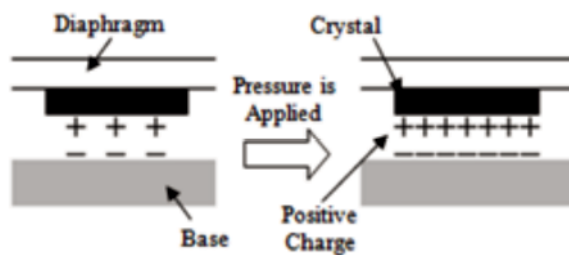
Fig 9. Sensor de presión Piezoeléctricos (Nurul et al. 2015)
