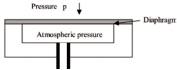
Fig. 7 Sensor de presión atmosférica. (Yunus et al. 2015)
