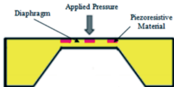
Fig. 8 Sensor de presión Piezorresistivo (Nurul et al. 2015)
