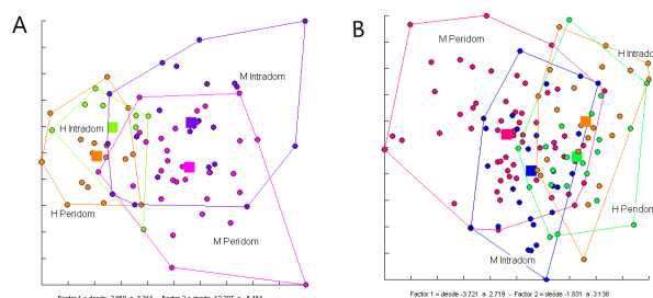
Figura 2: Análisis discriminante con las 4 variables antenales (A) y con las variables de conformación de la cabeza (B) de T. infestans colectados en pre tratamiento con insecticidas (2006) en intra y peridomicilio. Peridom: Peridomicilio, Intradom: Intradomicilio, H: Hembras, M: Machos. Fuente: Elaboración propia.
