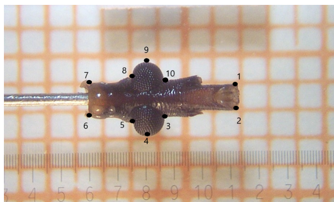
Figura 1: Vista ventral de la cabeza de Triatoma infestans con los 10 landmarks tipo II tomados para los análisis morfométricos. Los números indican el orden de captura de los landmarks. Fuente: Elaboración propia.
