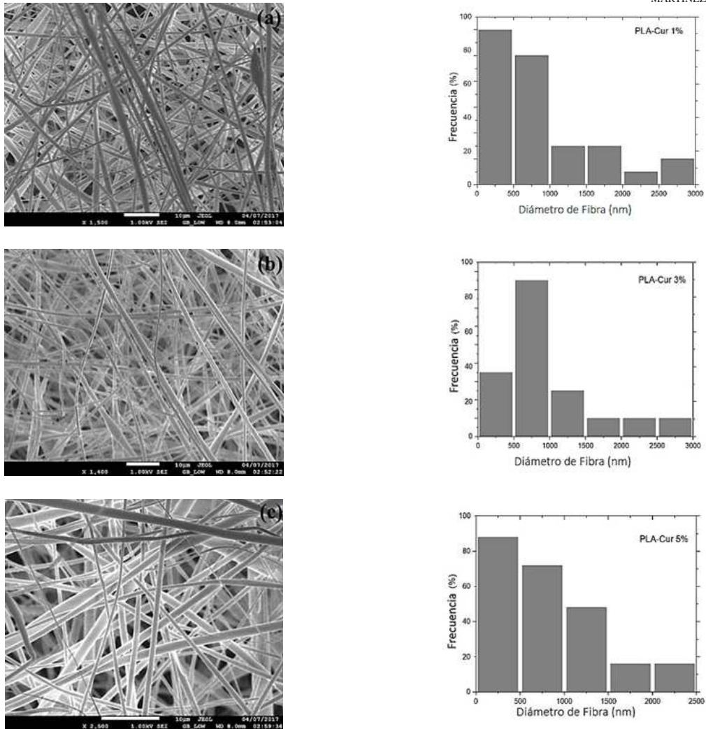
Figura 3: Imágenes SEM de PLA-Cur (a) 1%, (b) 3%, (c) 5%. Fuente: Elaboración propia.
