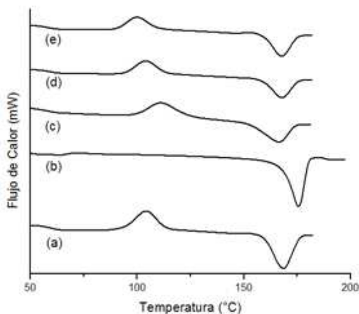
Figura 6: Curvas de calorimetría diferencial de barrido de (a) PLA, (b) Cur y PLA-Cur con concentraciones de (c) 5%, (d) 3%, (e) 1%. Fuente: Elaboración propia.
