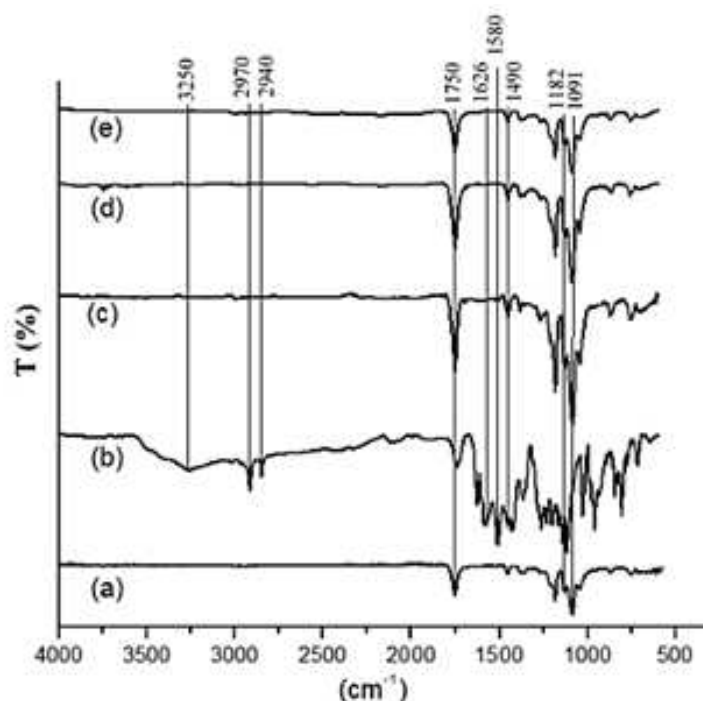
Figura 4: Espectro FTIR (a) PLA, (b) Cur y PLA-Cur con concentración de (c) 5%, (d) 3%, (e) 1%. Fuente: Elaboración propia
